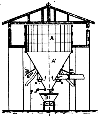
Fig. 12. — Séchoir Welkner.
